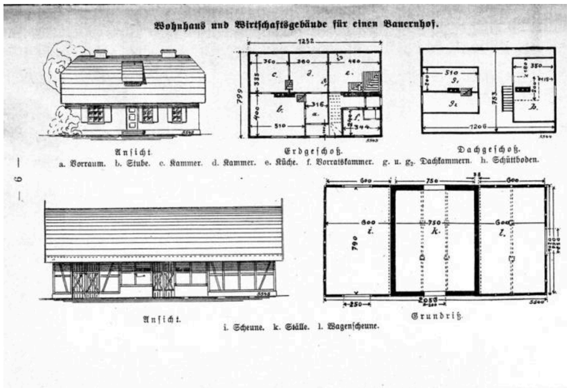
Seite 9 der Broschüre mit Ansicht und Grundriß für einen in Kurland zu errichtenden Bauernhof. Latvijas Nacionālā bibliotēka, CC0 1.0
